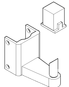
BOTTOM HINGE & BOX CAM
